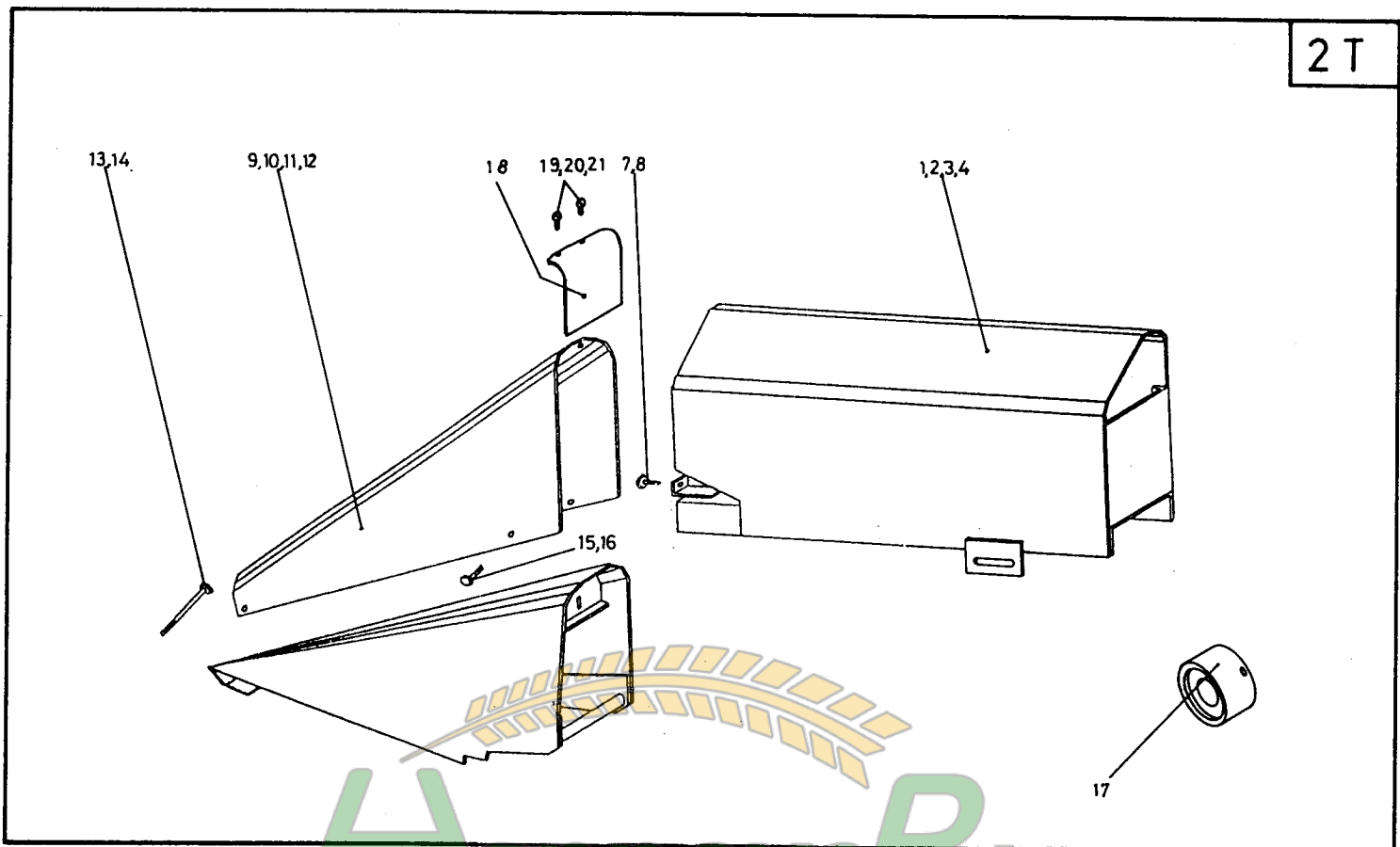
Außenkarosserieerhöhung - zweiteilig - Bildtafel 2T
